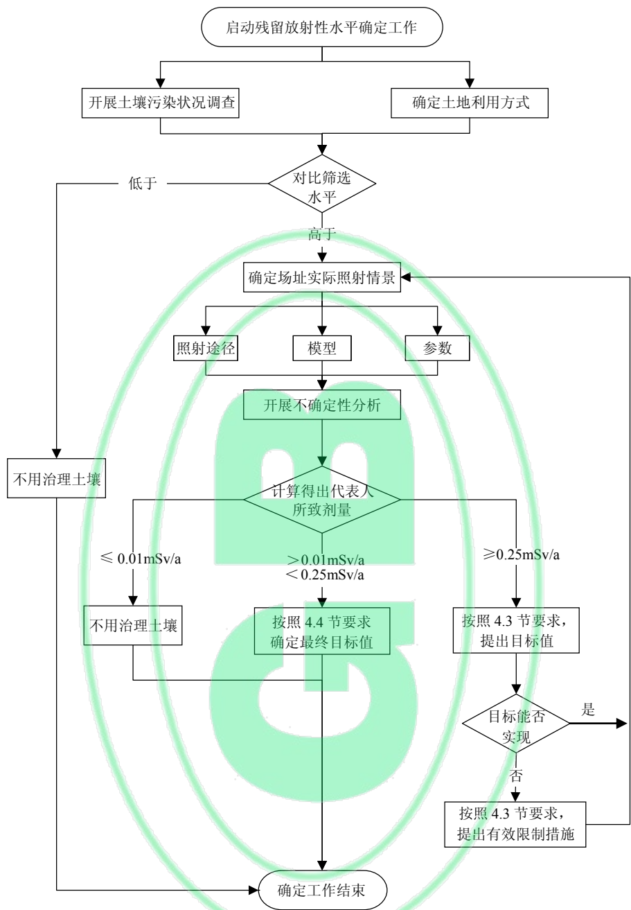
图 1 退役场址土壤中残留放射性水平确定的工作流程图
